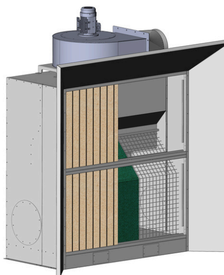
Ventilator oben mittig Auslass nach rechts
